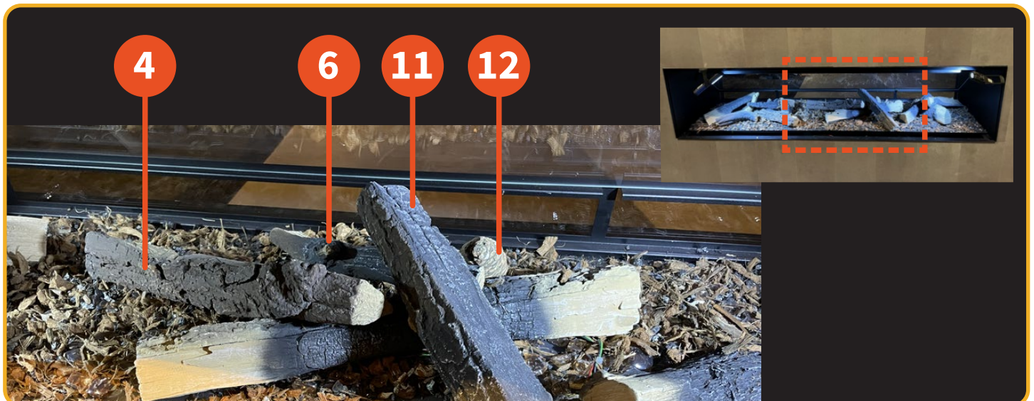
Afb. C.H | 6. Plaats de stammen in het middendeel zoals aangegeven
