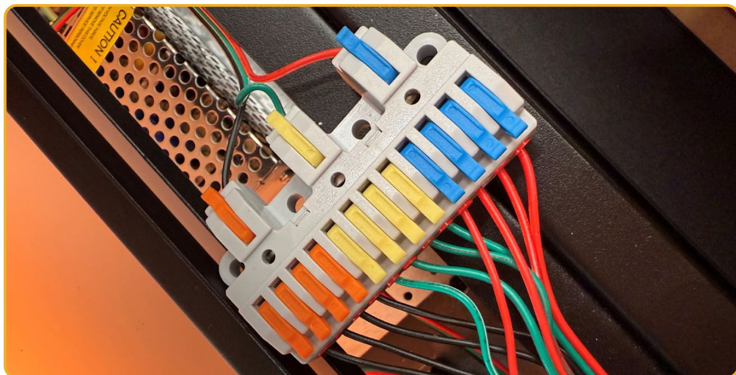
Afb. C.C | 2. Sluit kabels aan op lasklemmen
