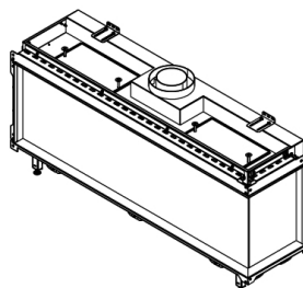
SUMMUM 140 CL
