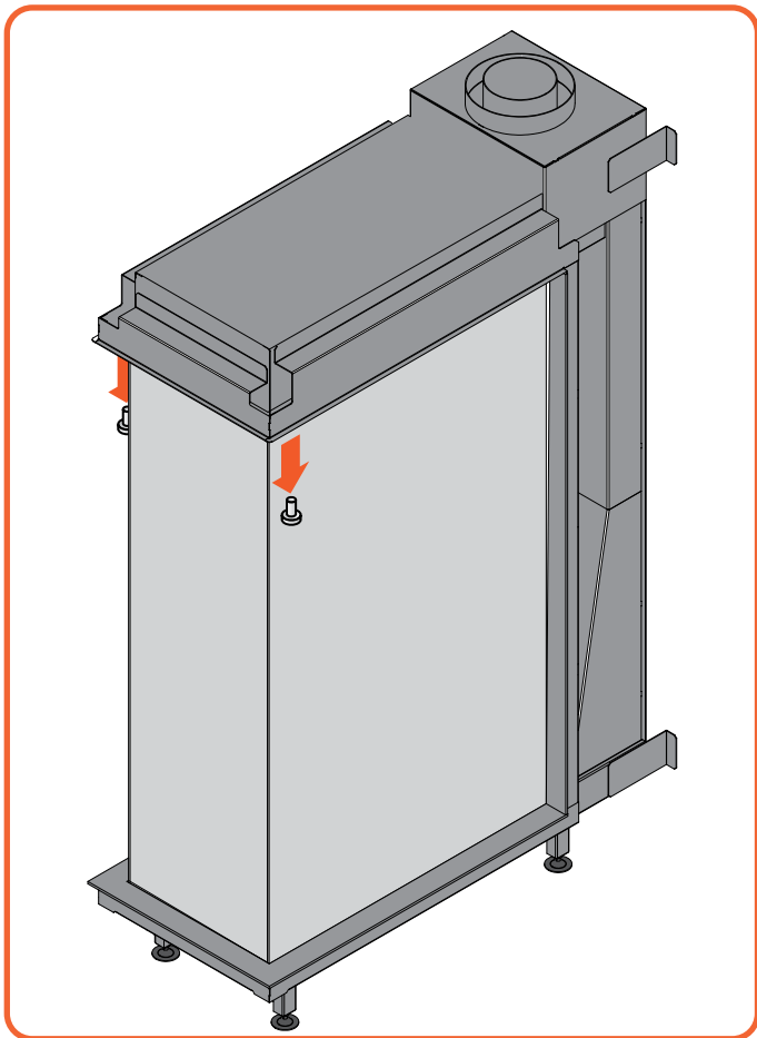
Figure 10.2 | Obere Blende abschrauben
