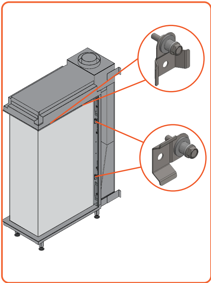
Figure 10.6 | Glashalterungen drehen
