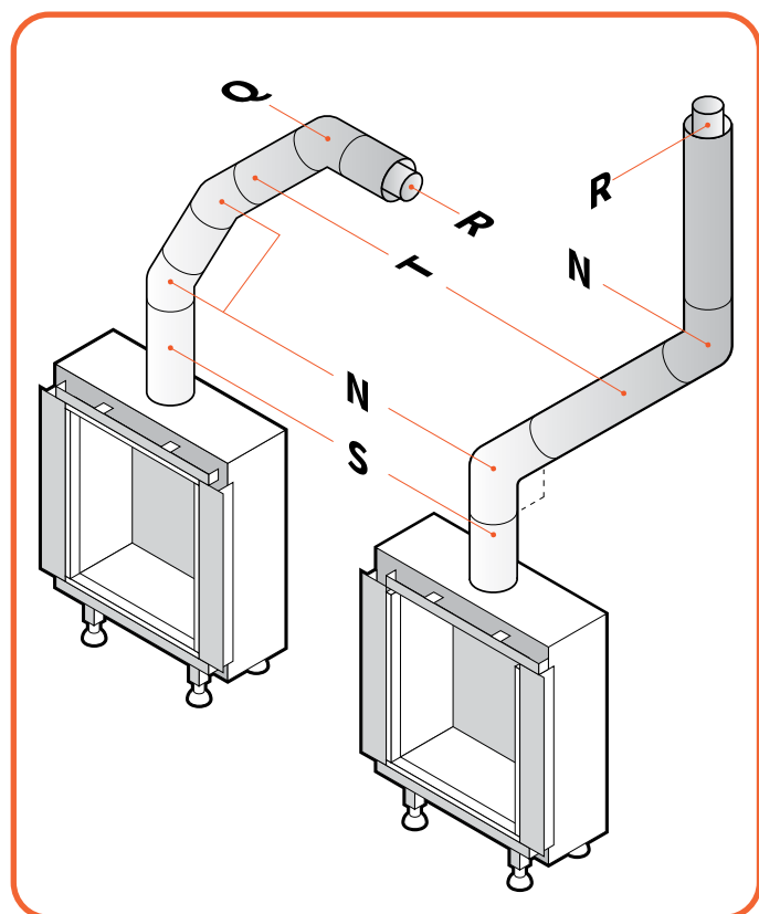
Figure 7.8 | Beispiele für Rauchrohrbögen
