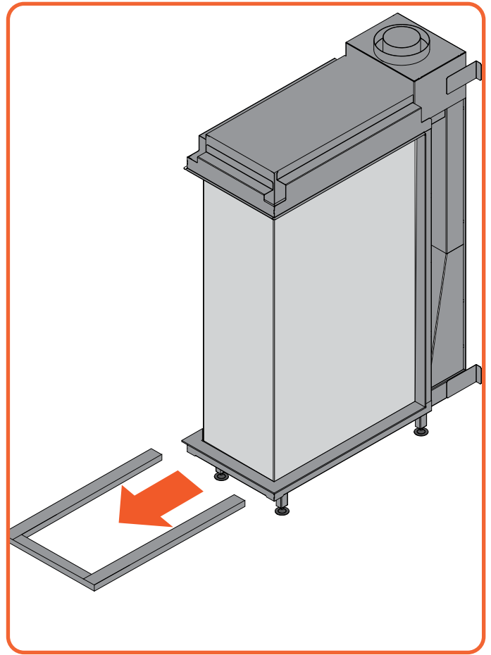
Figure 10.5 | Untere Blende entfernen
