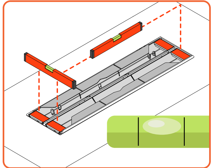
Figure 5.3 | Stellen Sie sicher, dass der Brenner waagrecht ist
