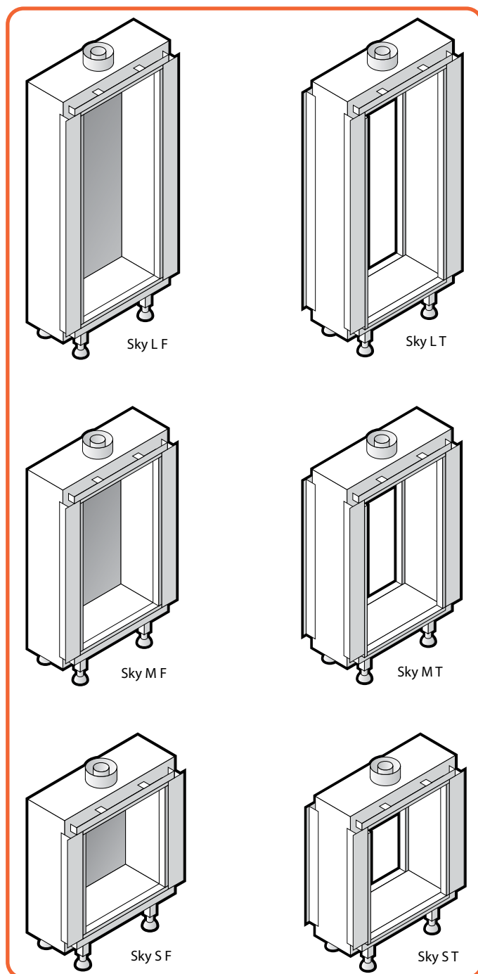
Figure 9.1 | Isometrische Ansicht Sky Modelle
