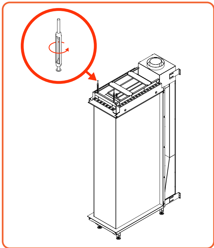
Figure 6.1 | Spannschlösser zur Befestigung des Kamins an der Decke
