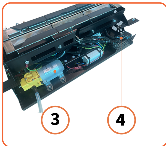
Figure 11.2 | Position von Befüllpumpe und Kraftstoffpumpe
