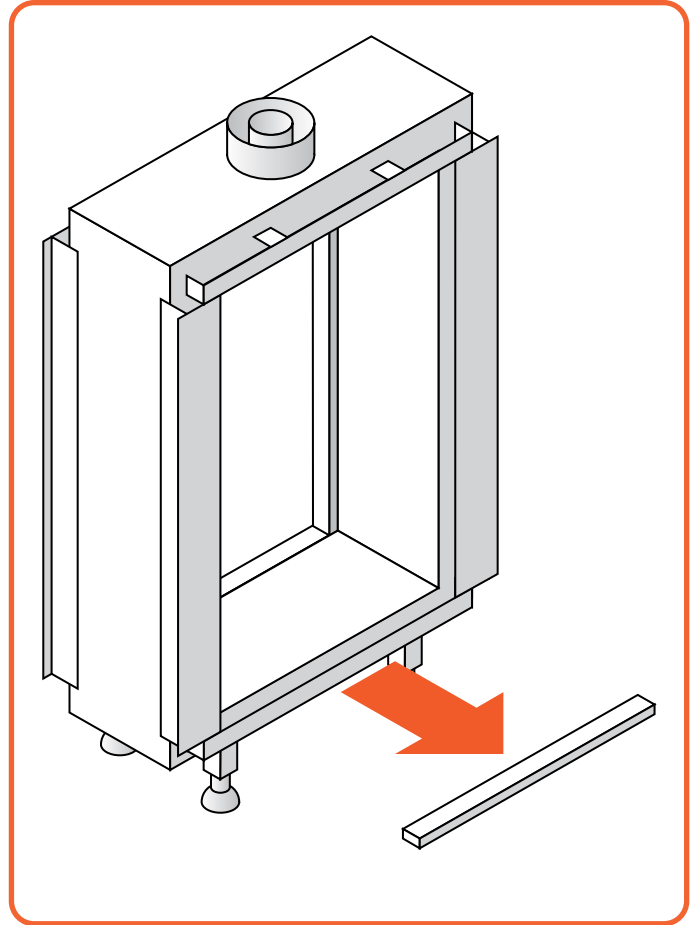
Figure 9.5 | Untere Blende entfernen
