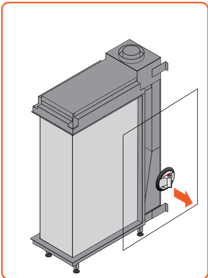
Figure 10.7 | Heben Sie das Glas vorsichtig aus dem Kamin
