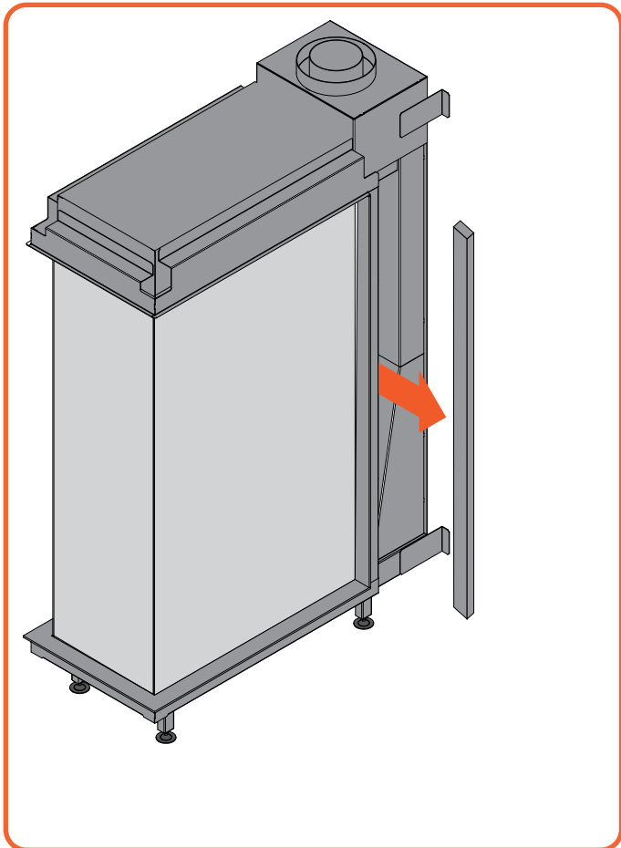
Figure 10.4 | Seitliche Blenden entfernen
