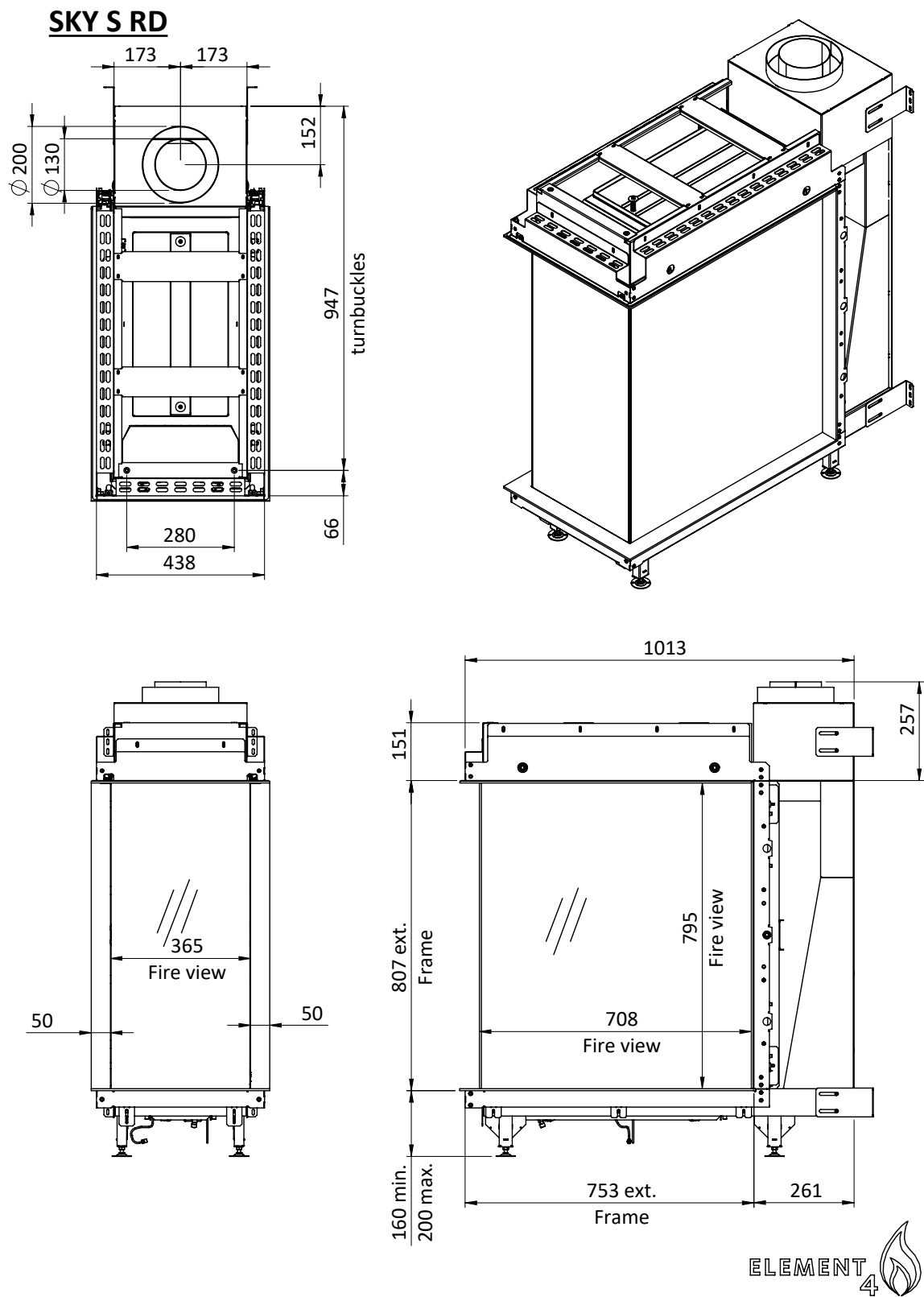
Figure G.A | Technische Zeichnung von Sky S RD
