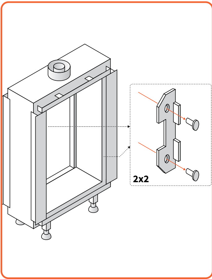
Figure 9.10 | Glas-Halterungen entfernen
