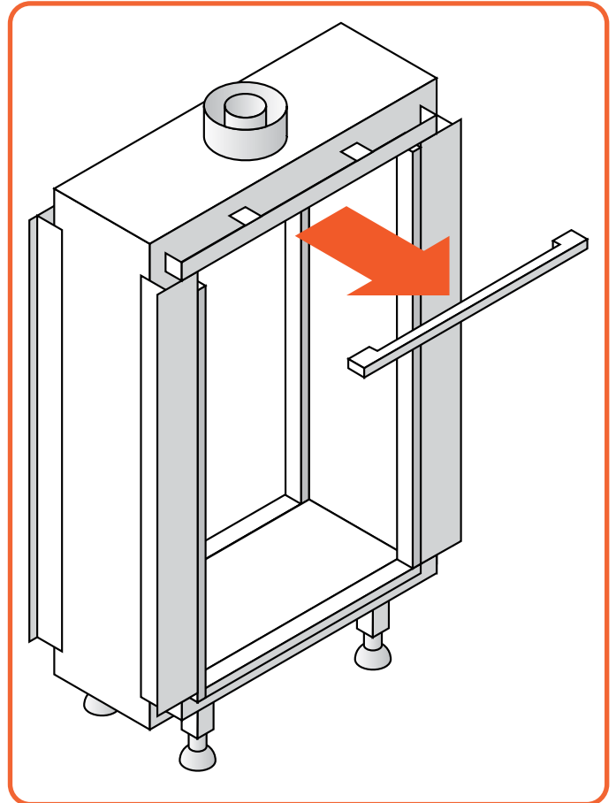
Figure 9.3 | Obere Blende entfernen
