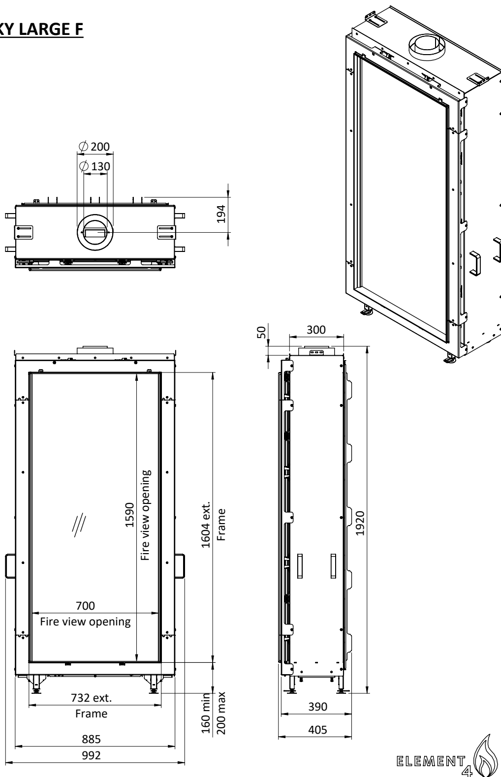
Figure F.A | Technische Zeichnung von Sky L F
