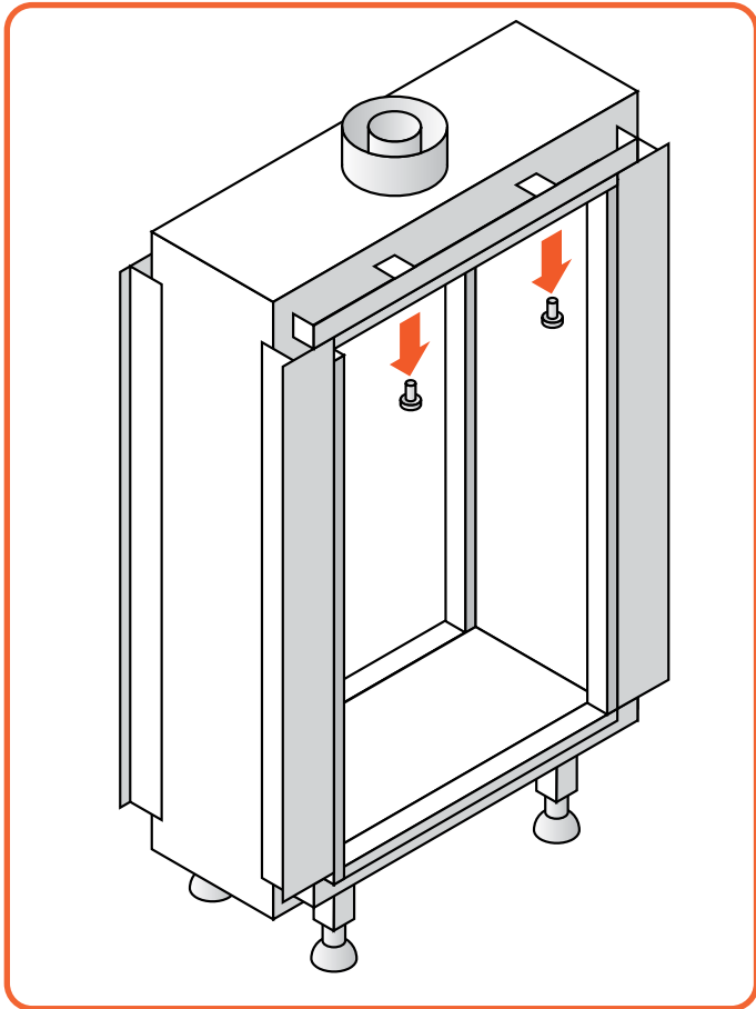
Figure 9.2 | Schrauben der oberen Blende entfernen
