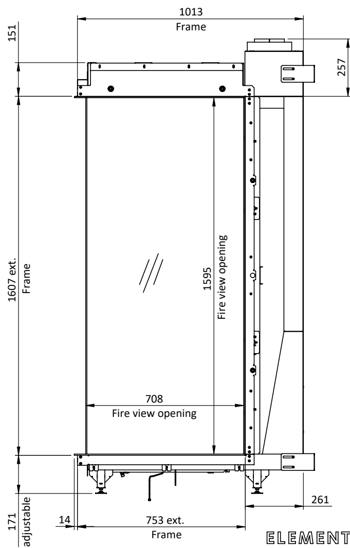
Figure G.C | Technische Zeichnung von Sky L RD
