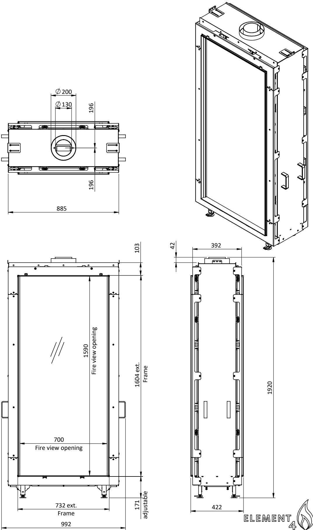
Figure F.B | Technische Zeichnung von Sky L T
