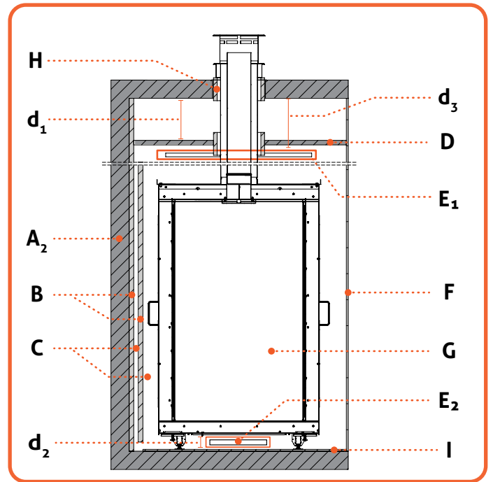
Figure 6.5 | C11: Abgassituation Brennbare Materialien
