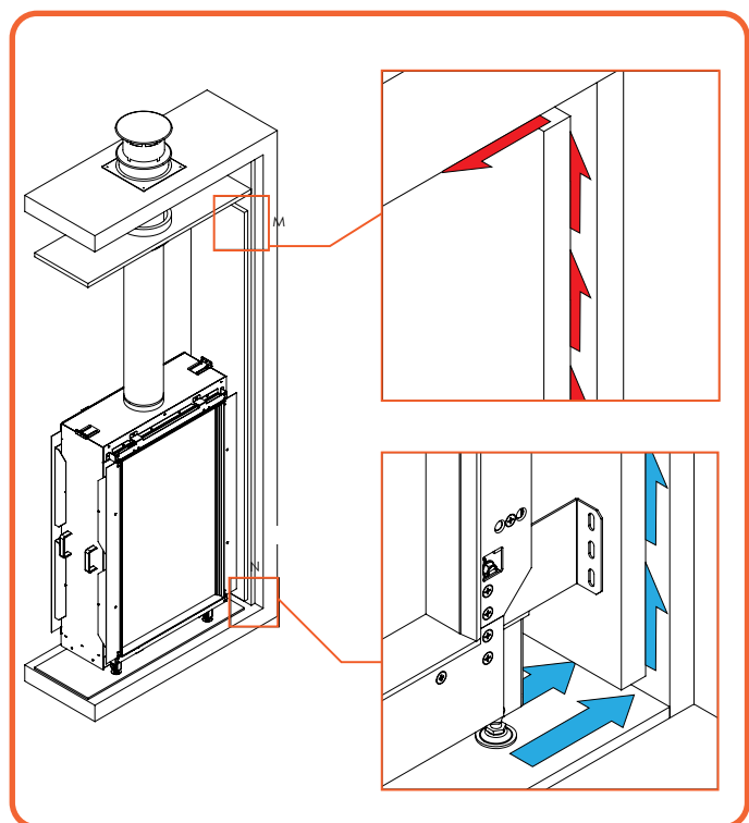
Figure 6.6 | Luftstrom zwischen Wandabdeckungen
