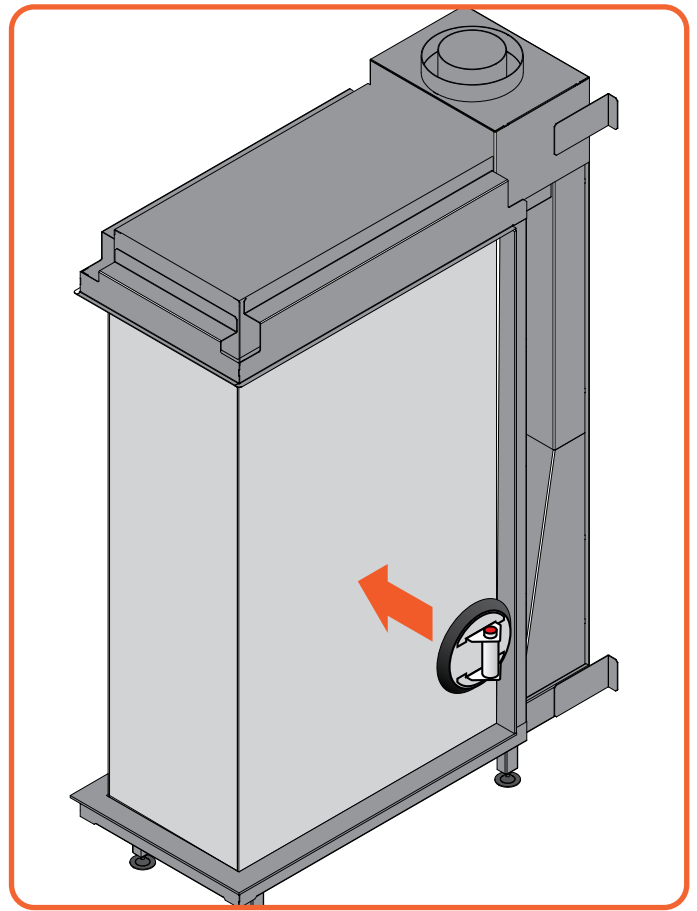
Figure 10.8 | Saugnapf auf das Glas setzen
