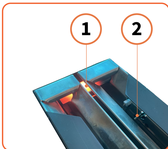
Figure 11.1 | Position von Zünder und Thermoelement
