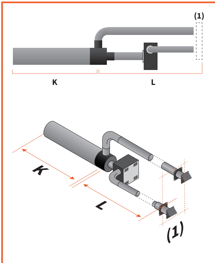
Afbeelding 3.12 - Opbouwsysteem 2.2
