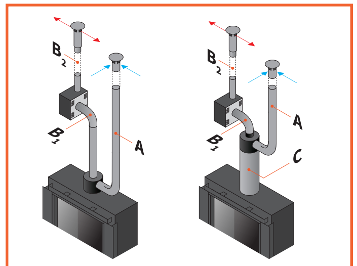
Afbeelding 1.6 - Verticale uitmondungen
