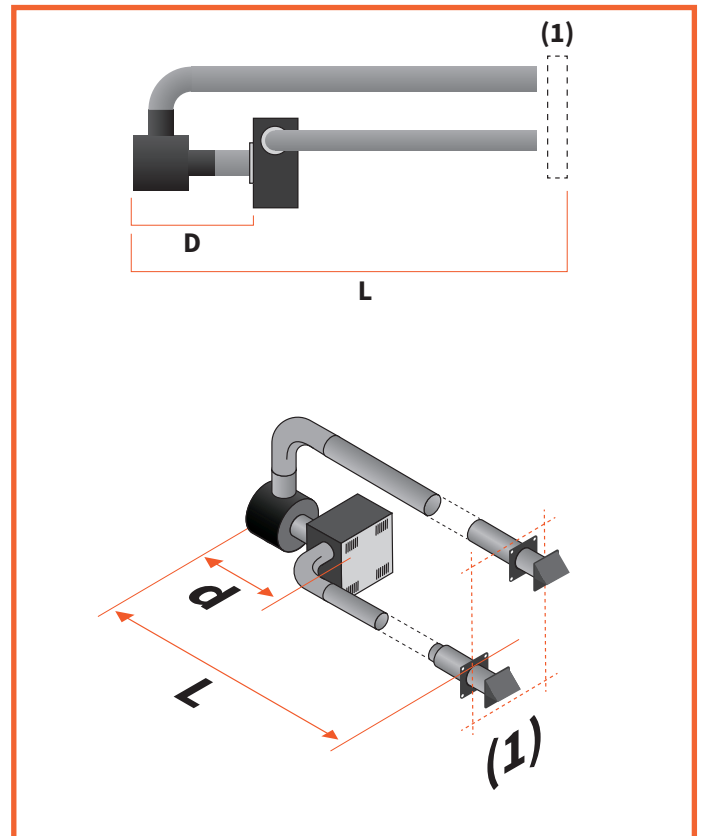
Afbeelding 3.10- Opbouwsysteem 1
