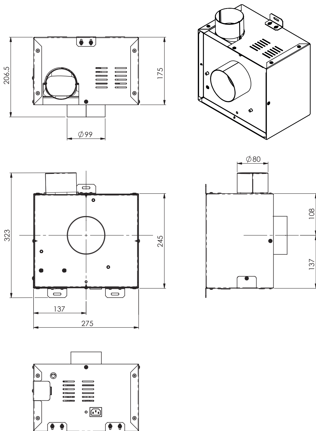
Afbeelding 7.2 - Dimensies PowerFan MkII
