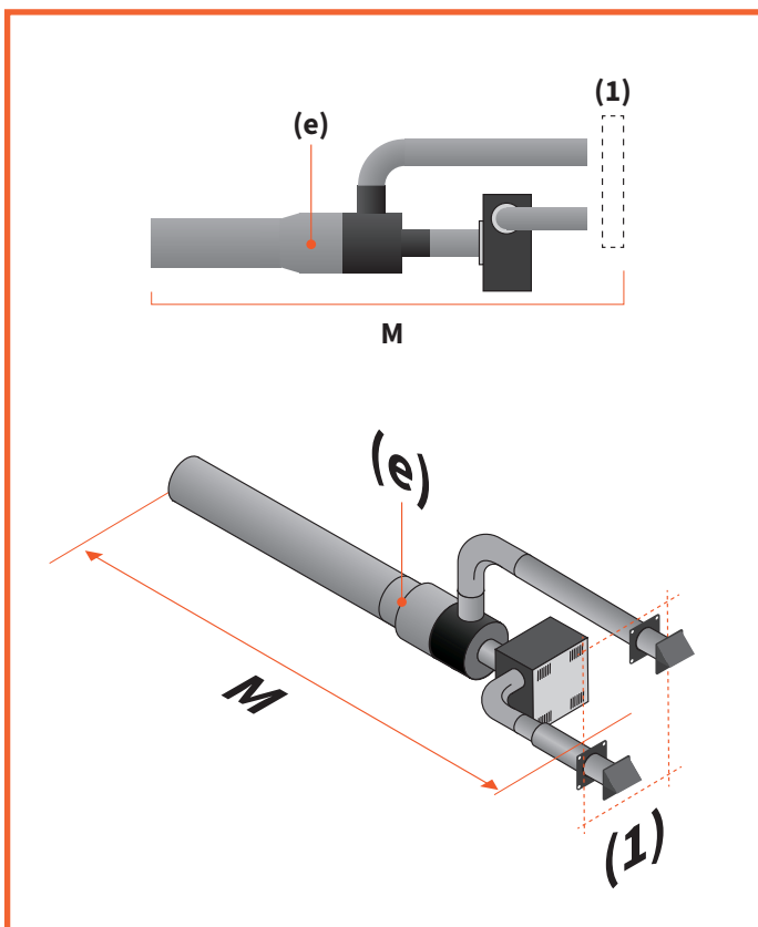
Afbeelding 3.13 - Opbouwsysteem 2.3
