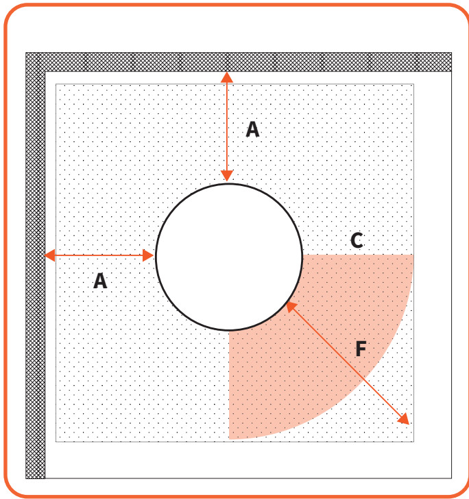
Afb. 6.1 Afstanden tot brandbare apparaten (boven)
